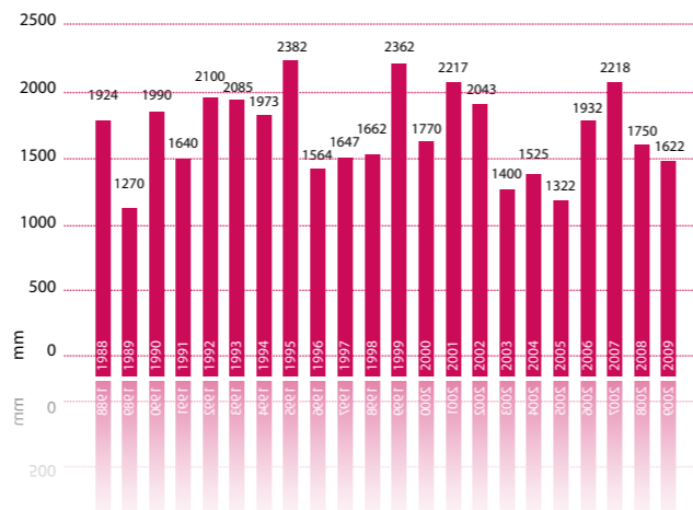
PRÉCIPITATIONS ANNUELLES SUR LES 22 DERNIÈRES ANNÉES
