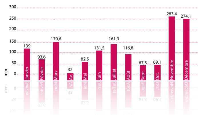
PRÉCIPITATIONS DE L'ANNÉE 2009
