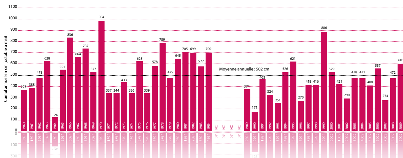
ENNEIGEMENT ANNUELLE AU COURS DES 50 DERNIÈRES ANNÉES
